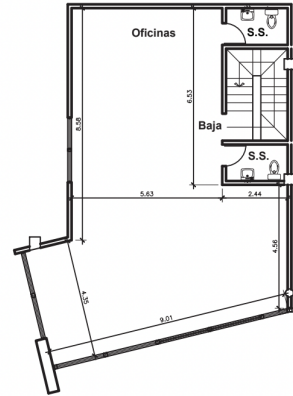
PLANTA ALTA
