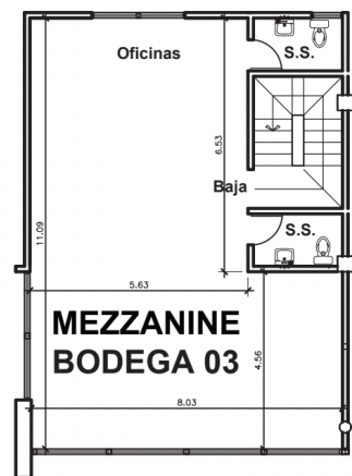
PLANTA ALTA
