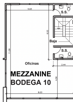
PLANTA ALTA
