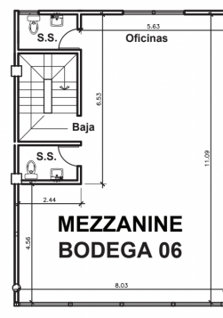
PLANTA ALTA
