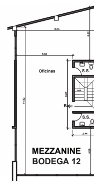
PLANTA ALTA
