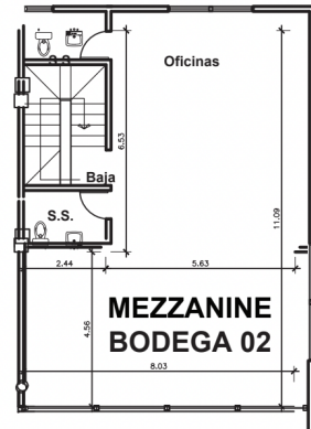
PLANTA ALTA
