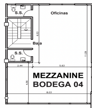
PLANTA ALTA
