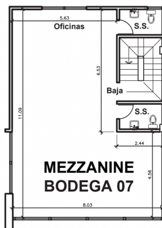
PLANTA ALTA
